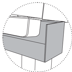
Profilo gronda strutturale / Structural gutter profile
